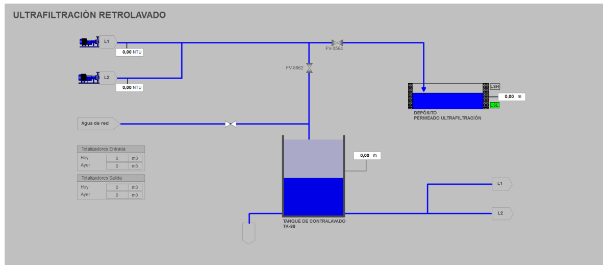
Figura 24. Pantalla SCADA Ultrafiltración Retrolavado
