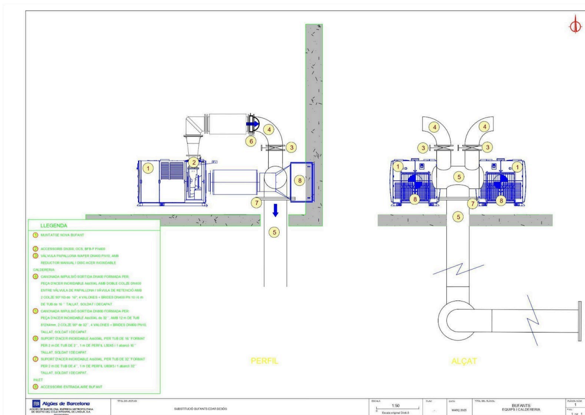
Fig. 5 Esquema aportació impulsió de les bufants.
